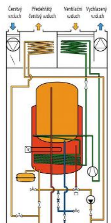
Obr. 4 - Detail ventilačního tepelného čerpadla F470 (A)
