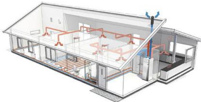
Obr. 3 • Schéma rovnotlakového větrání v rodinném domě [4]
